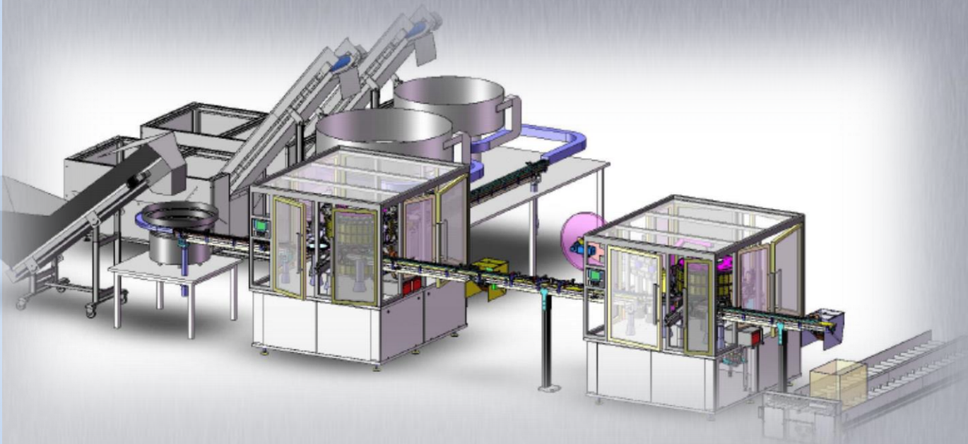
kontinuierliche Montage-Maschine im Rundläufer-Prinzip zur Verschluss-Deckel-Montage
